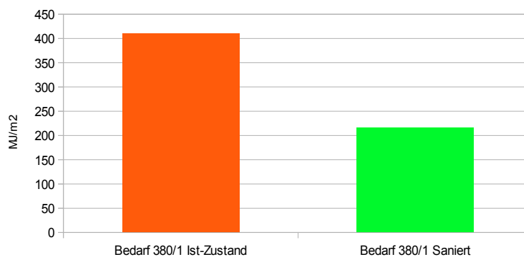
Energieeinsparung Westtrakt nach SIA 380/1
